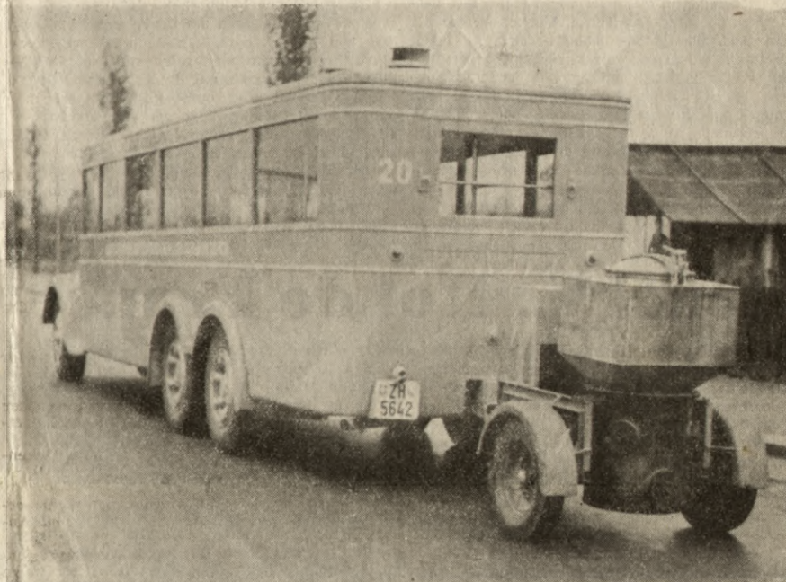
Holzvergaser auch für die Autobusse der Städte. Um der völligen Lahmlegung des Autobusverkehrs zu steuern, sind nun in Zürich, dessen Straßenbahnverwaltung über einen gewaltigen Autobuspark verfügt, erfolgreiche Versuche mit dem neuen Holzgasgenerator angestellt worden und es besteht berechnete Aussicht, daß schon in nächster Zeit sämtliche Autobuslinien der Straßenbahn mit Holzkohlengas gefahren werden. (ATP)
